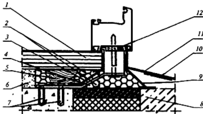
Рисунок А.4 - Узел нижнего примыкания оконного блока, подоконника и слива к проему слоистой стены с эффективным утеплителем
