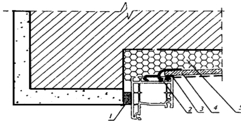
Рисунок А.13 - Узел бокового и верхнего примыкания оконного блока к проему стены с четвертью и отделкой внутреннего откоса панелями
