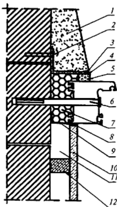
Рисунок А.2 - Узел бокового примыкания оконного блока к проему без четверти в стене из кирпича и отделкой внутреннего откоса облицовочной панелью
