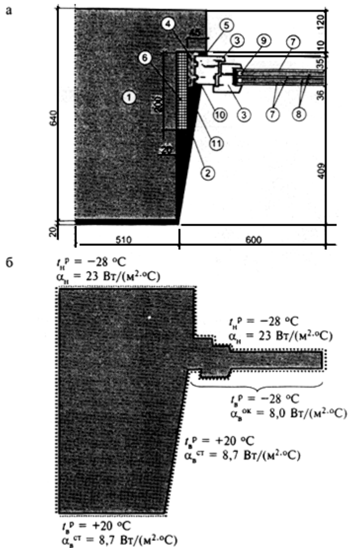
Рисунок Г.2 - Расчетная схема (а) и схема задания граничных условий (б) узла примыкания оконного блока к оконному проему
