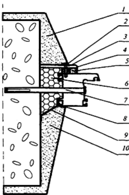
Рисунок А.7 - Узел бокового примыкания оконного блока к проему без четверти в стене из ячеистобетонных блоков с отделкой фасада, наружных и внутренних откосов штукатурным раствором
