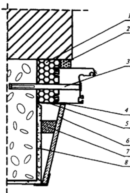
Рисунок А.6 - Узел бокового примыкания оконного блока к проему с четвертью в стене из ячеистобетонных блоков (плотностью 400-450 кг/м 2 с облицовкой кирпичом и отделкой внутреннего откоса панелью
