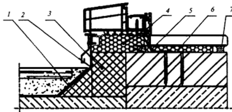
Рисунок А.11 - Монтажный шов в нижнем узле примыкания коробки балконной двери
