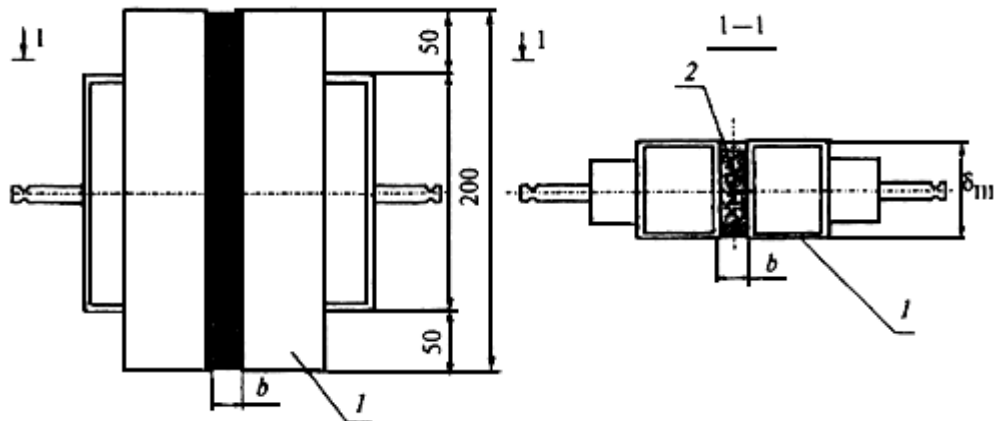
Рисунок 4 - Схема приспособления для испытания монтажных швов на деформационную устойчивость
