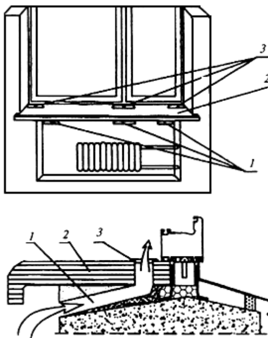
Рисунок А.17 - Схема нижнего узла примыкания с каналом подачи теплого воздуха от нагревательного прибора к оконному блоку
