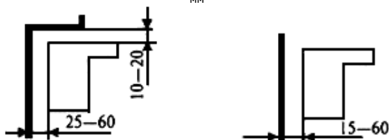
Рисунок 2 - Размеры монтажных зазоров (швов) при установке оконных блоков из различных материалов по ГОСТ 23166
