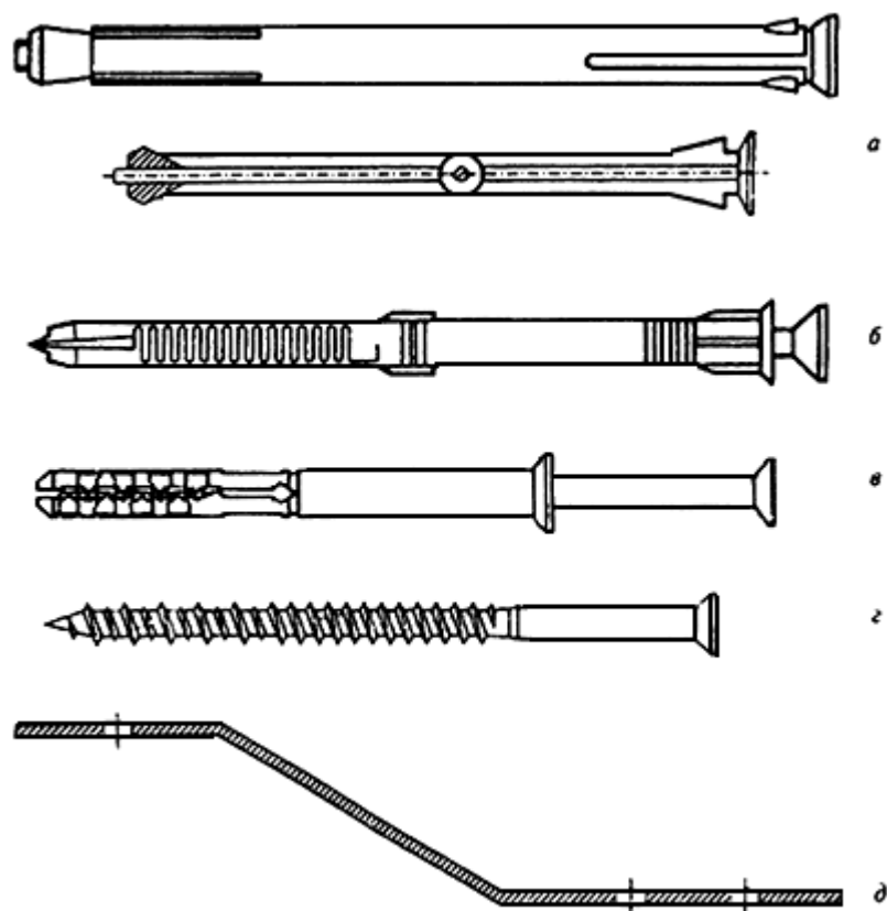
Рисунок Б.1 - Примеры крепежных элементов
