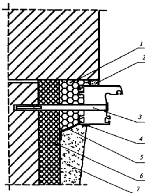
Рисунок А.1 - Узел бокового примыкания оконного блока к проему с четвертью в стене из кирпича, с отделкой внутреннего откоса штукатурным раствором
