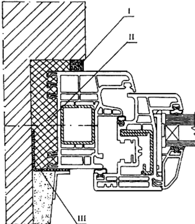
Рисунок 1 - Принципиальная схема монтажного шва
