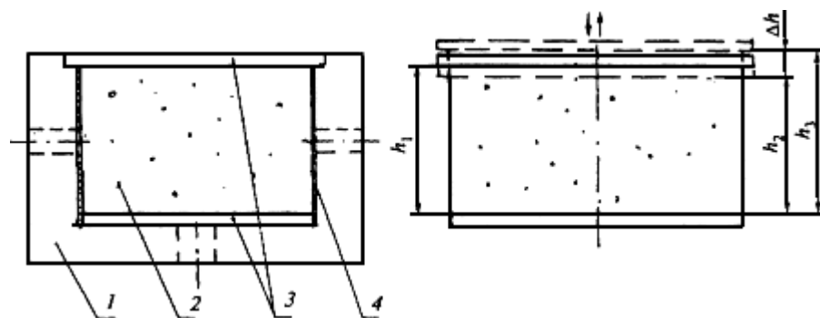
Рисунок 4а - Схема устройства для подготовки образцов и испытания пенного утеплителя на деформационную устойчивость
