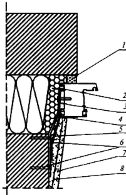
Рисунок А.3 - Узел бокового примыкания оконного блока к проему с четвертью слоистой стены из кирпича с эффективным утеплителем и отделкой внутреннего откоса штукатурным раствором
