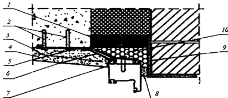
Рисунок А.5 - Узел верхнего примыкания оконного блока к перемычке из стального уголка в проеме многослойной стены с облицовкой кирпичом
