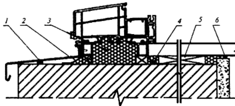
Рисунок А.12 - Монтажный шов в нижнем узле примыкания оконной коробки, подоконника и отлива в проеме однослойной стены
